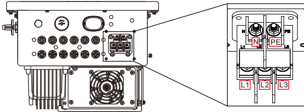
图5.18 逆变器交流端子
