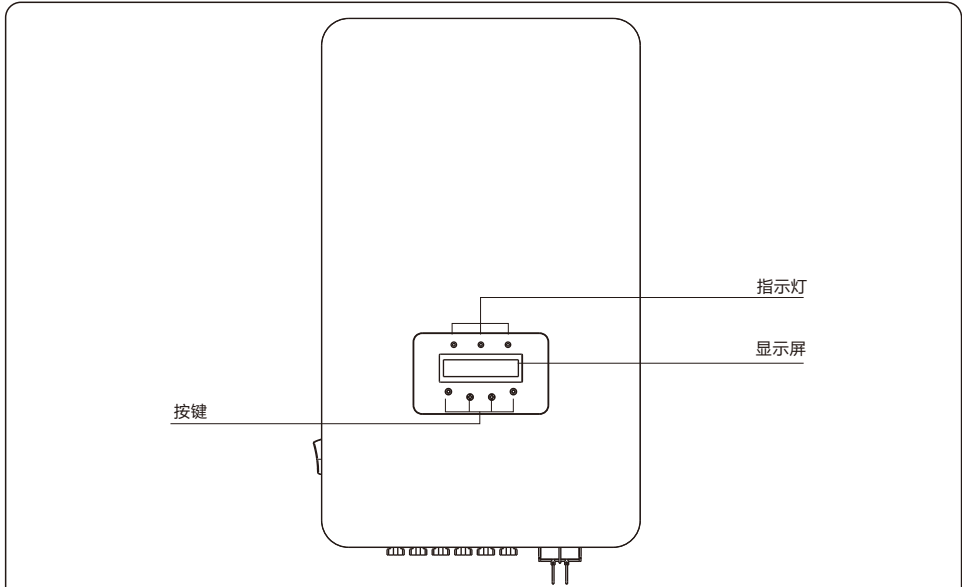
图1.1 逆变器正视图
