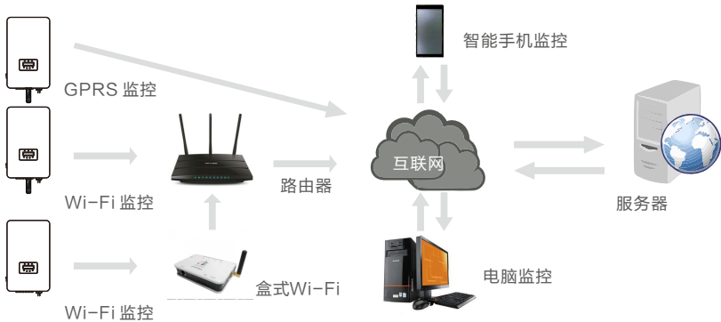
图5.19 逆变器通信方式示意图
