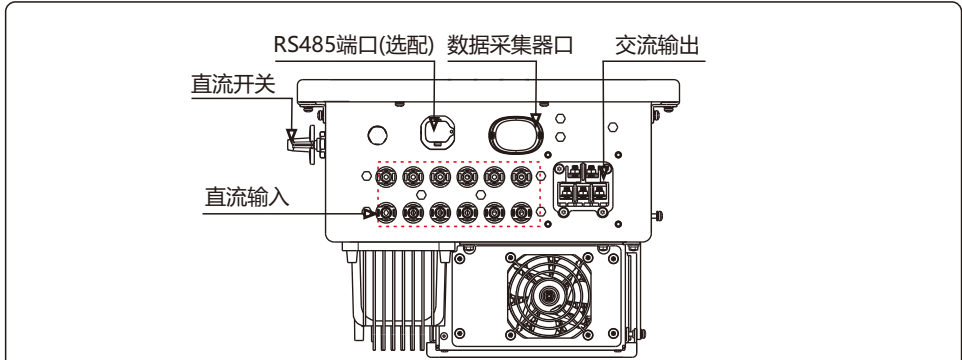
图1.2 逆变器底面视图
